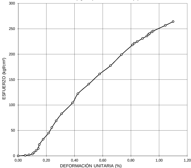
ESFUERZO (Kgf/cm 2 ) VS.DEFORMACIÓN (%)
